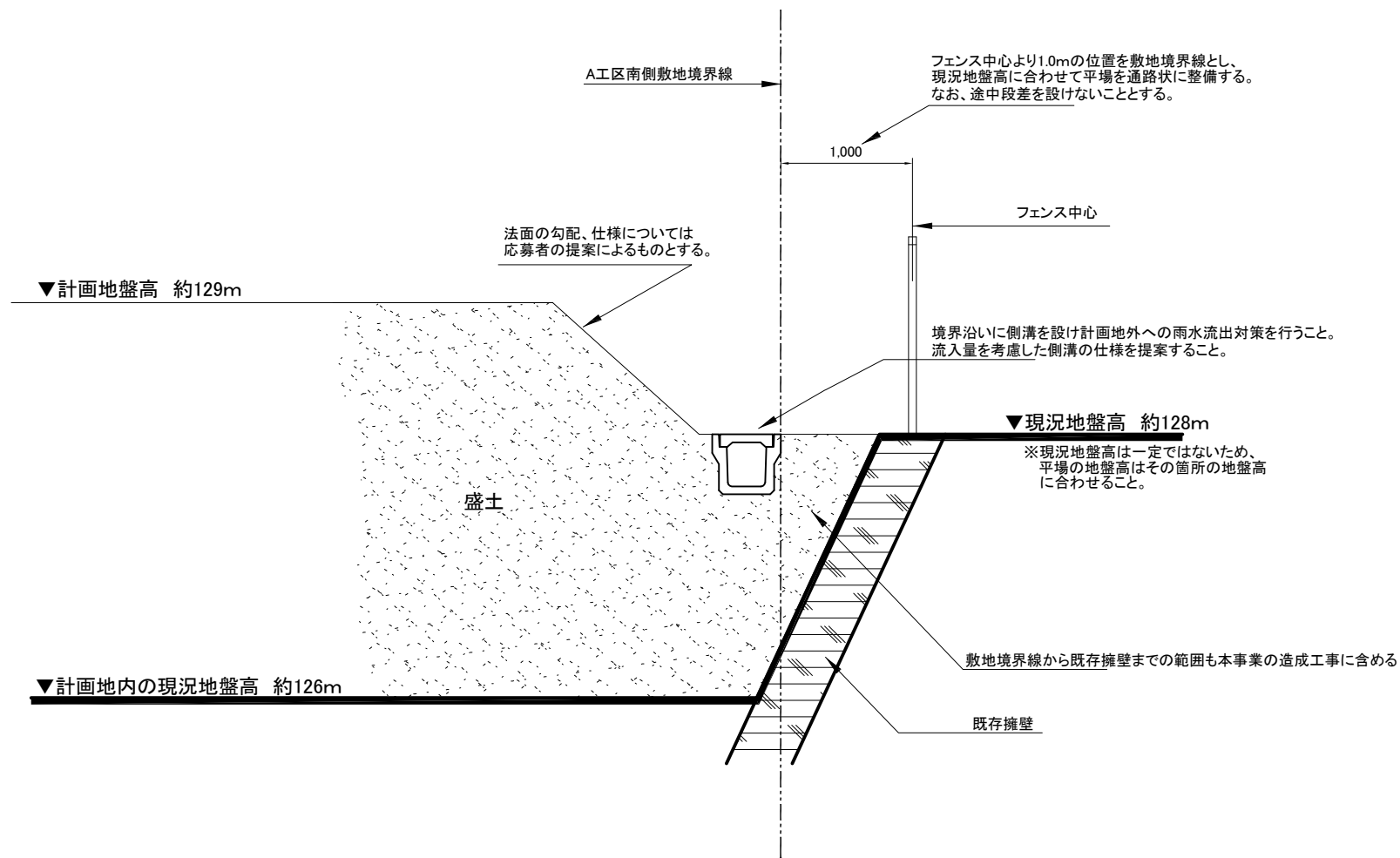
A工区敷地南側境界線の造成計画の考え方
